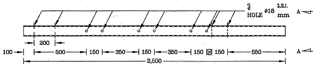
การติดตั้งสวิตช์เปิดได้เมื่อมีไหลต ชนิด SF 6 SF 6 LOAD BREAK SWITCH INSTALLATION
