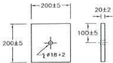
ขนาดแป้นรองมิเตอร์ 20x20 เซนติเมตร สำหรับยึดสายเข้า และออกจากมิเตอร์ สำหรับติดตั้งมิเตอร์ 1 เฟส ที่แผงจ่ายค่า
