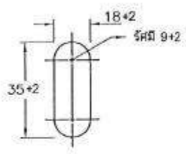
รายละเอียด A การเจาะรู \phi 18x35 มิลลิเมตร
