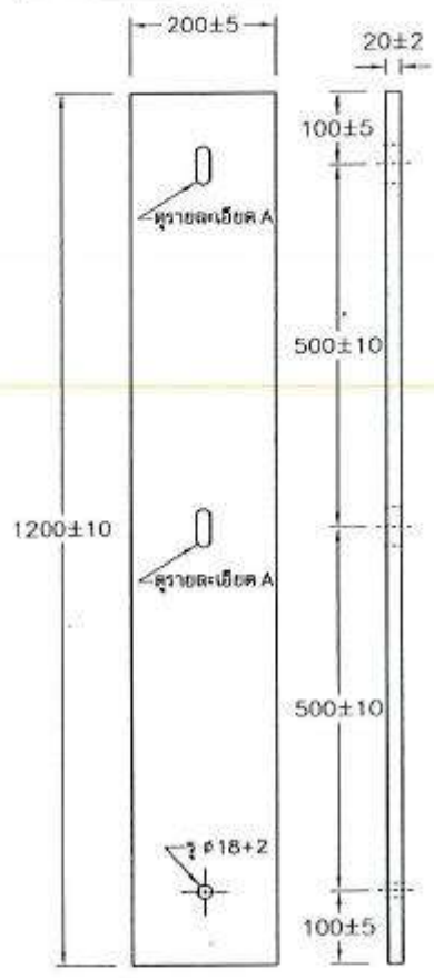
ขนาดแป้นรองมิเตอร์ 20x120 เซนติเมตร สำหรับมิเตอร์ 3-4 เครื่อง
