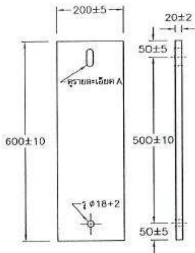
ขนาดแป้นรองมิเตอร์ 20x60 เซนติเมตร สำหรับมิเตอร์ 1-2 เครื่อง สำหรับรองรับมิเตอร์ที่ติดตั้งในตู้มิเตอร์
