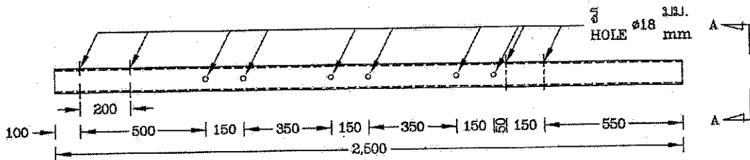
การติดตั้งสวิตช์เปิดได้เมื่อมีโหลด ชนิด SF 6 SF 6 LOAD BREAK SWITCH INSTALLATION
