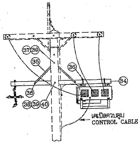
การติดตั้งสวิตช์เปิด-ปิดได้อิมโฟลด์ ชนิด SF 6 SF 6 LOAD BREAK SWITCH INSTALLATION
