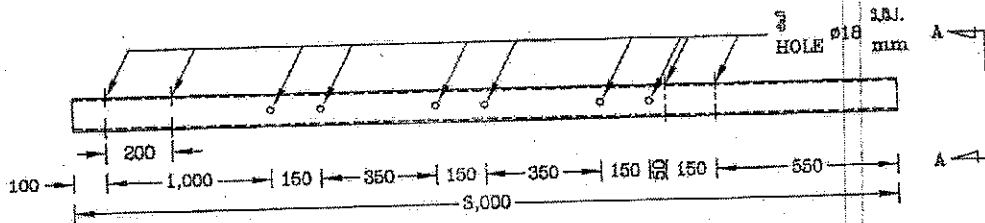
การติดตั้งสวิตช์เปิด-ปิดได้อิมโฟลด์ ชนิด SF 6 SF 6 LOAD BREAK SWITCH INSTALLATION
