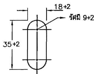
รูยึดสายเข้า A การเจาะรู 18x35 มิลลิเมตร
