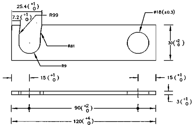
รายละเอียด D แผ่นเหล็ก 120x30x3 มม.
