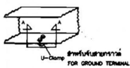
รายละเอียด A จุดต่อสายดิน DETAIL A GROUND TERMINAL
